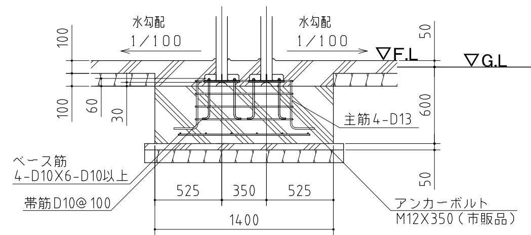
A-A' 断面
